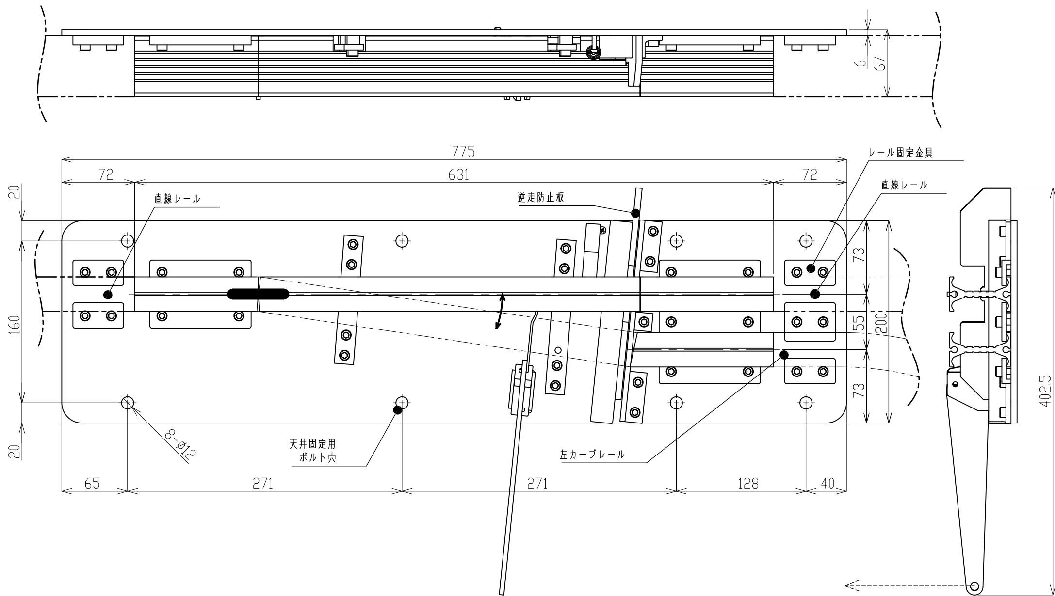
キャリー左分岐ユニット (28L92)
