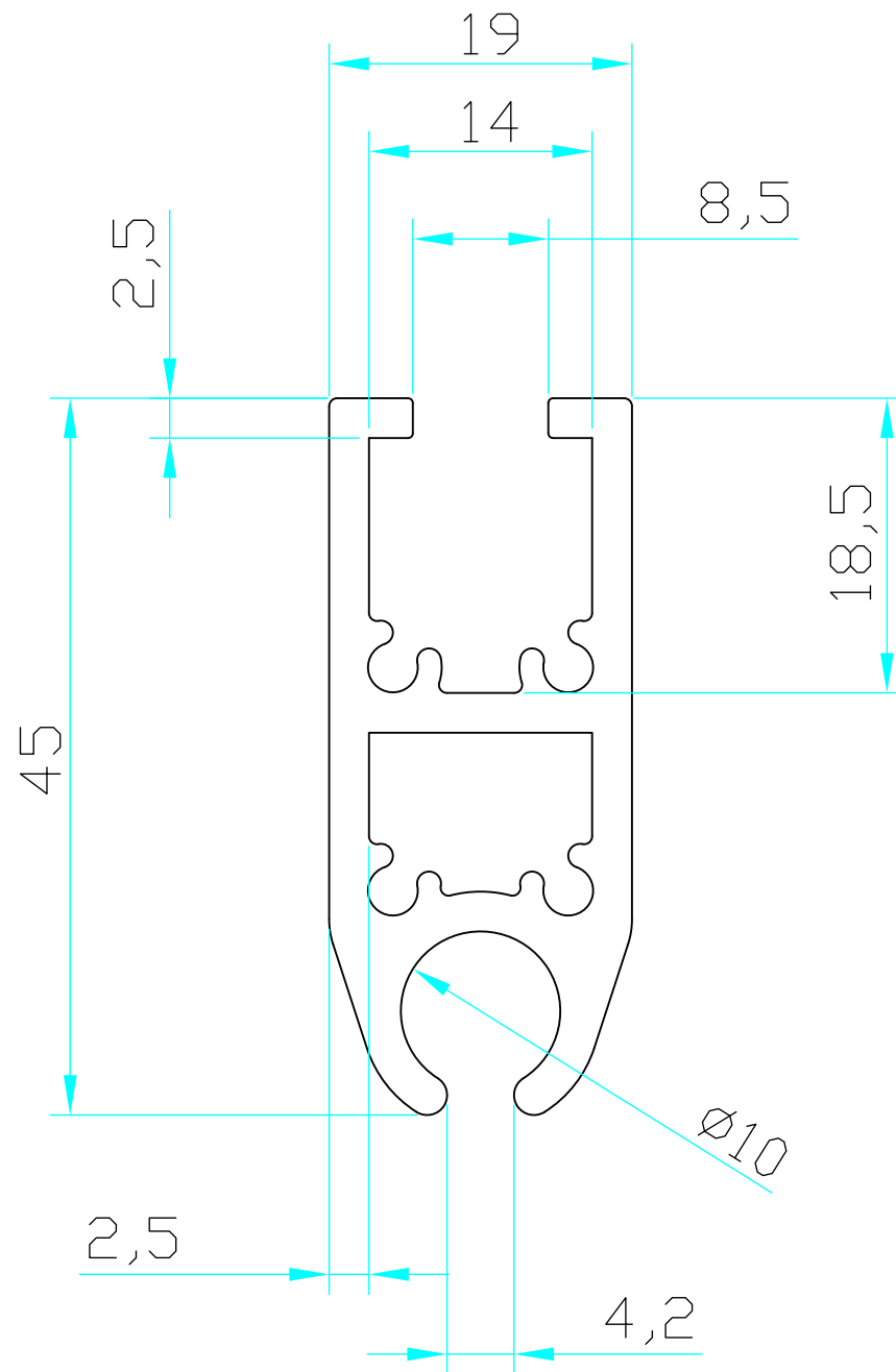
テンションバー AM型 (82L43)
