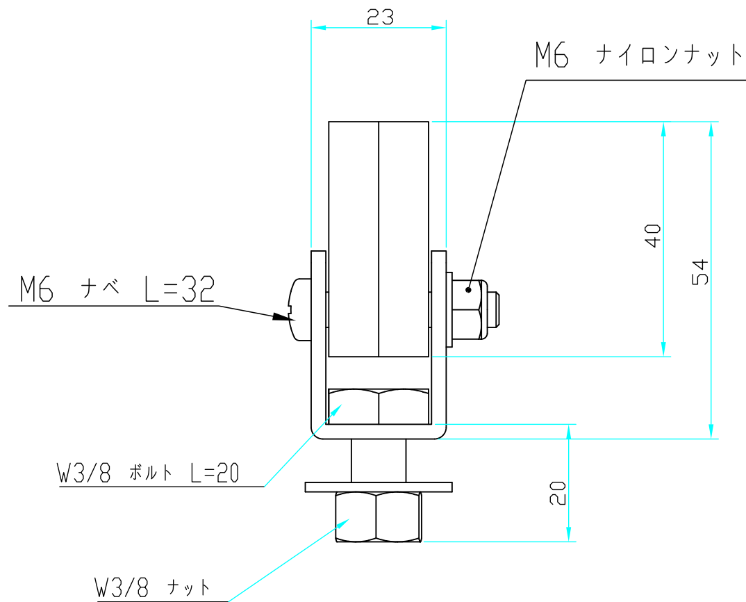
寸切りボルト取付金具 (00Y59)
