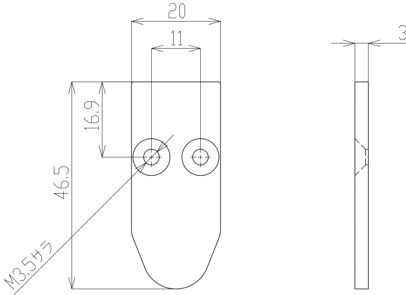
テンションバーAM型アルミキャップ (82T43)
