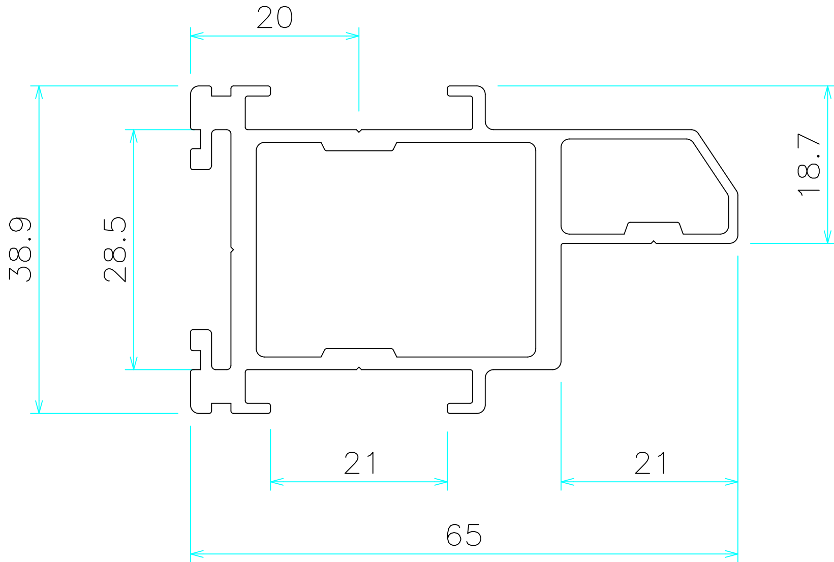
間仕切 サイドポール XG ----- (95S***)
