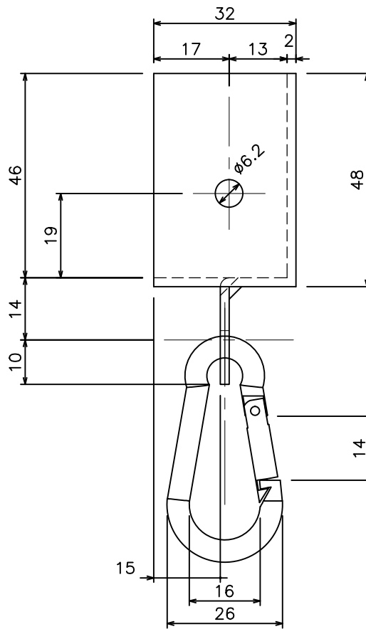
SG ステンキャップストップD (27T31D)
