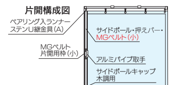
片開構成図
