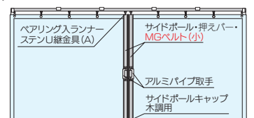
片開構成図
