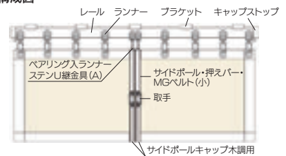
両開構成図
