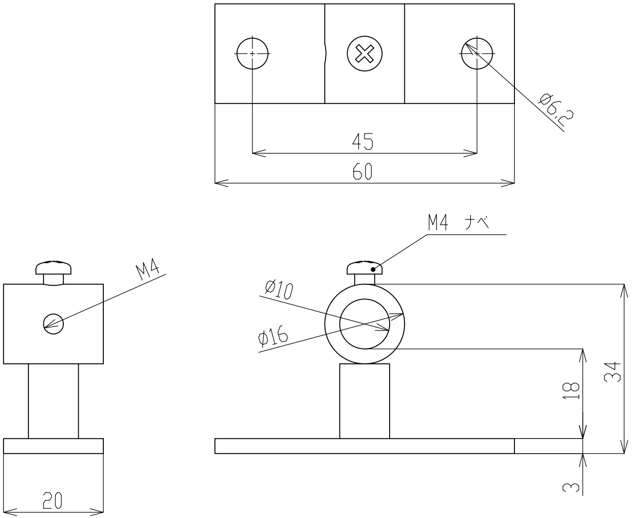
LBブラケット (9φ用) (77LB41)
