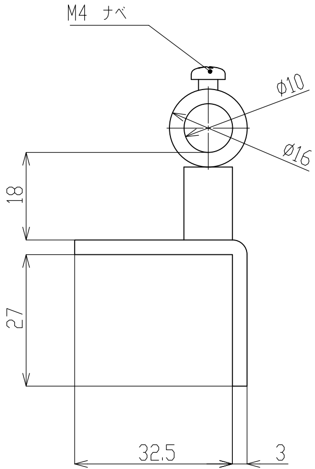
LBL型ブラケット (9φ用) (77LB42)
