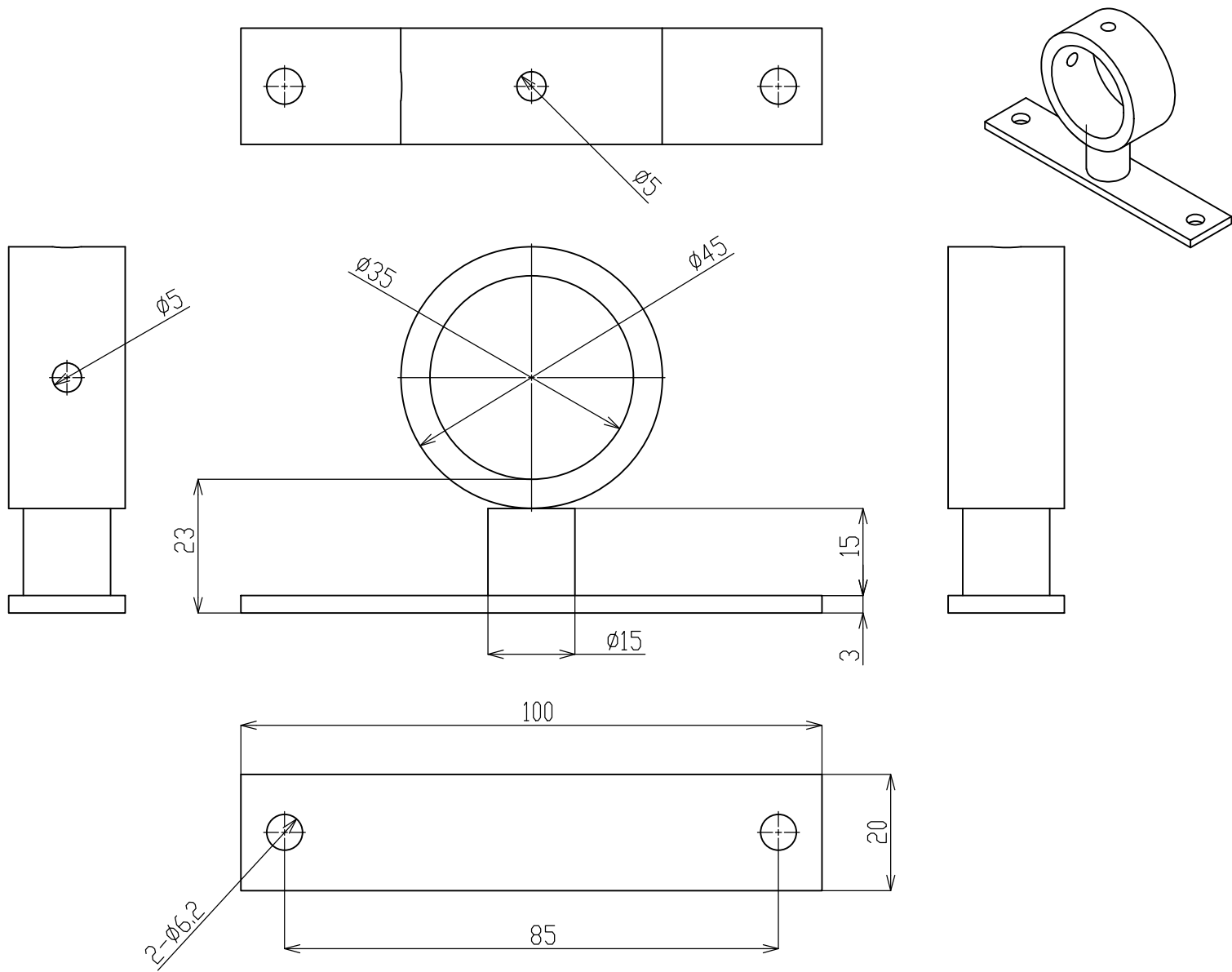
LBブラケット (34φ用) (79LB41)
