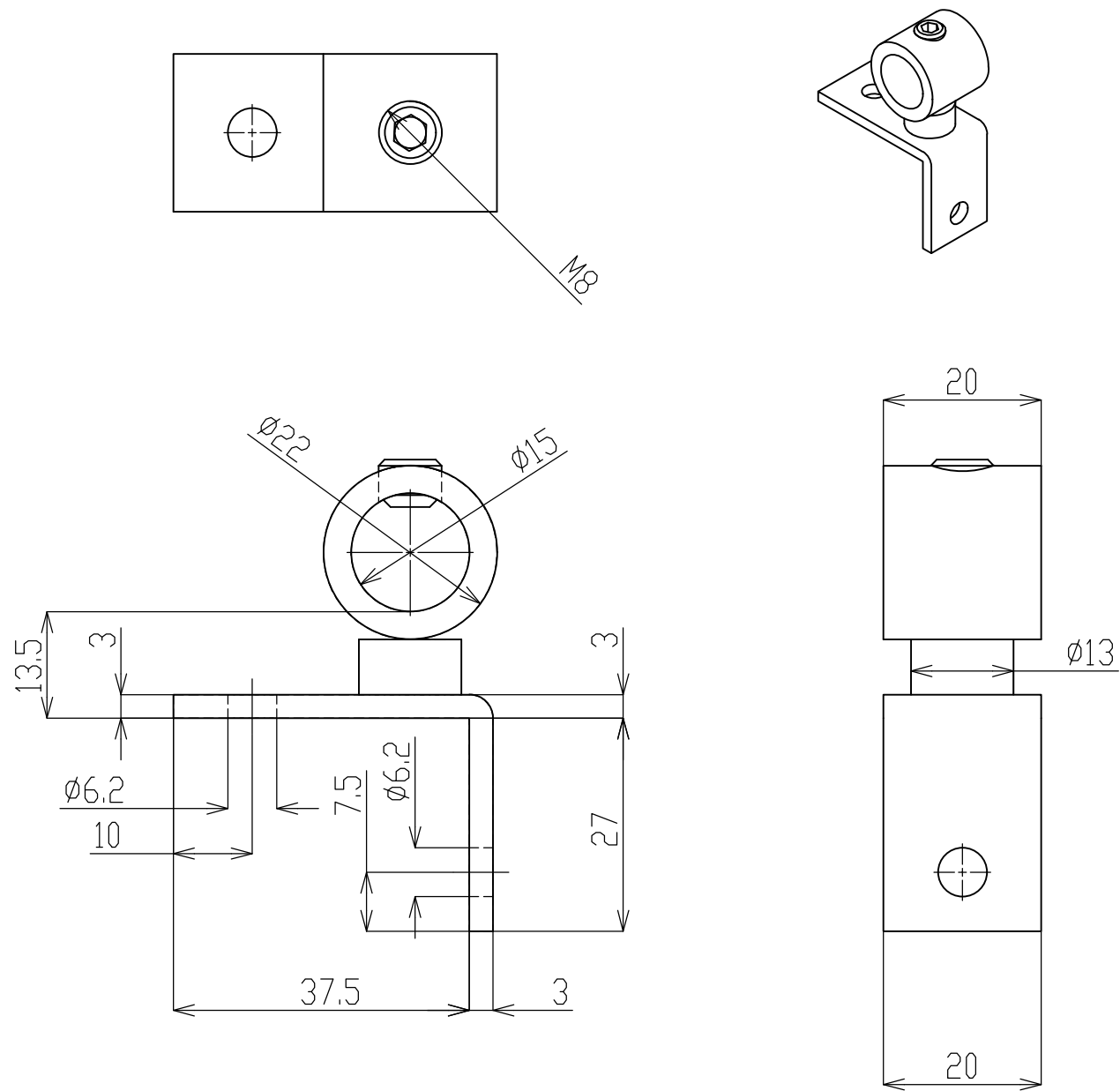
LB L型ブラケット (13φ用) (78LB42)
