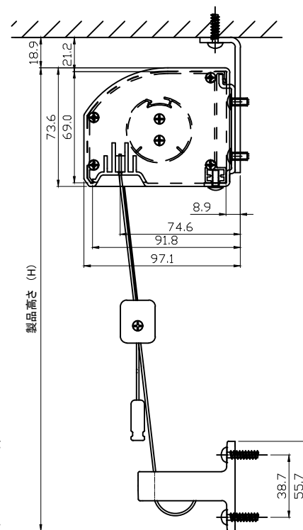
スリムブラケット
