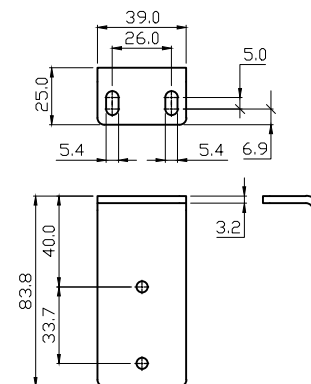
天井付金具
