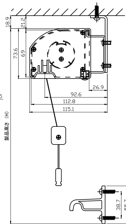
標準ブラケット
