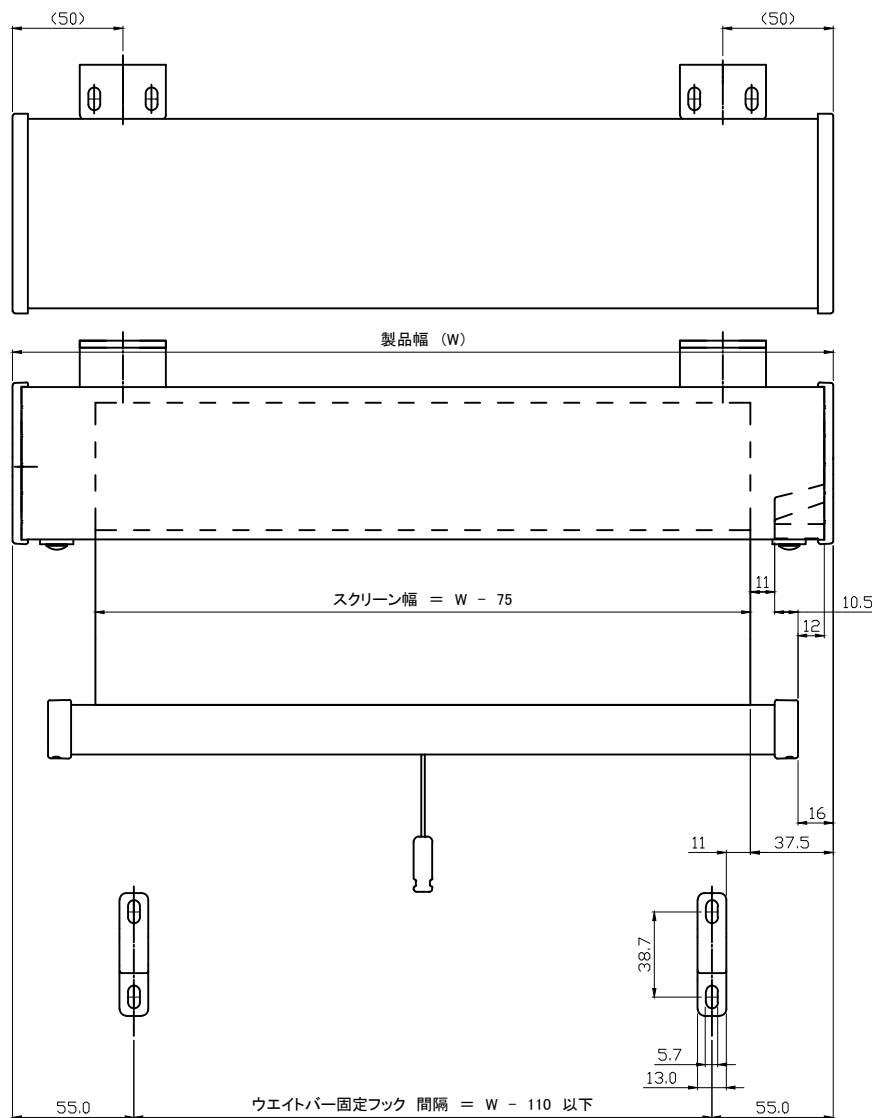
標準ブラケット
