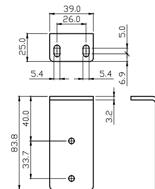
天井付金具
