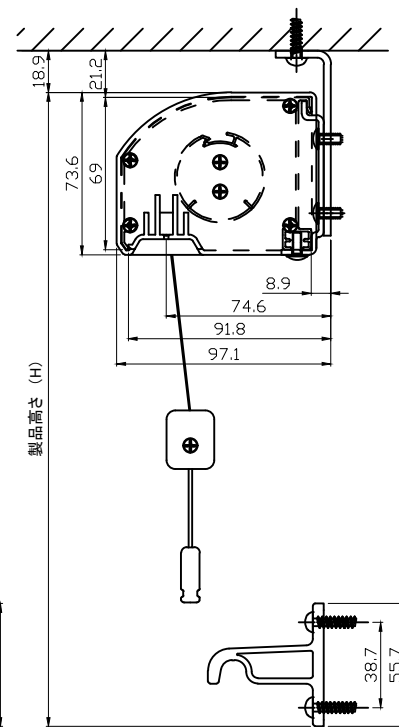
スリムブラケット
